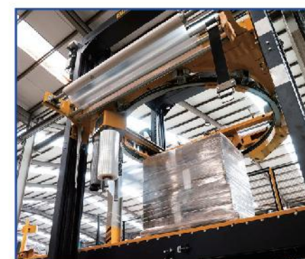
环轨式 Ring Wrapper
